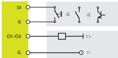
（开关量输入/输出接线图）
