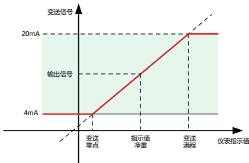
4-20mA输出计算模型(可类比单极性信号)
