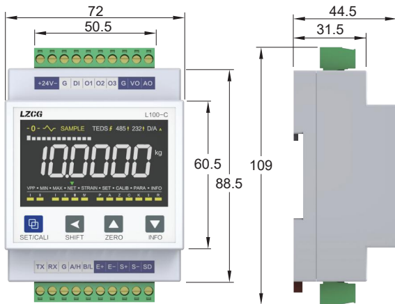
(侧视图)
