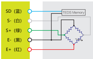
（传感器&TEDS接线图）
